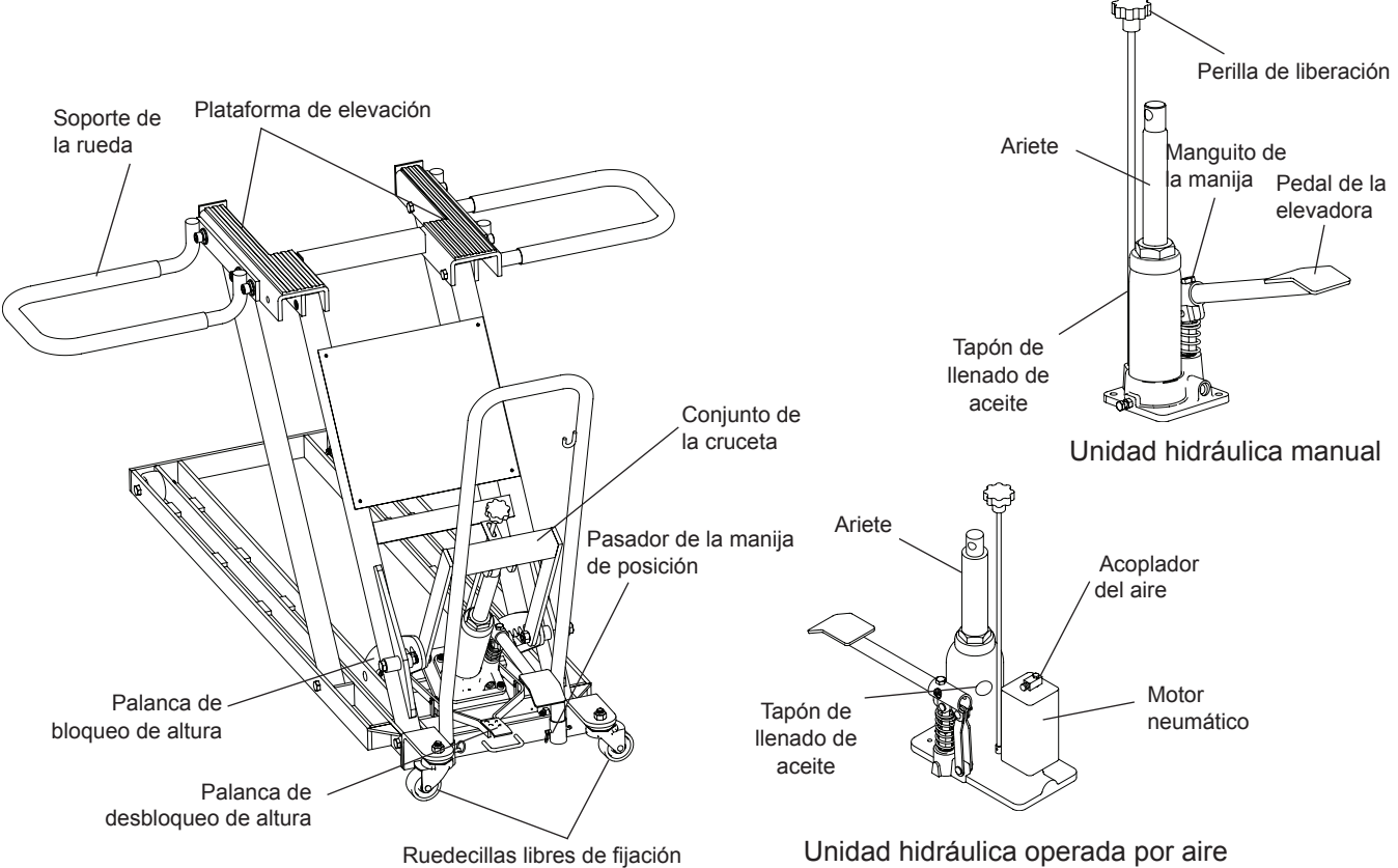
Figura 1: nomenclatura de los modelos T-5500/T-5501
