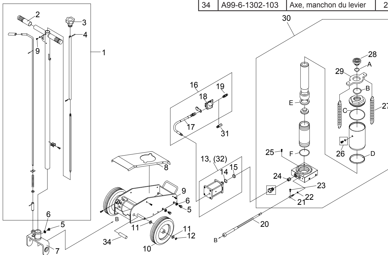
Figure 4 : Illustration des pièces de rechange du modèle 23991
