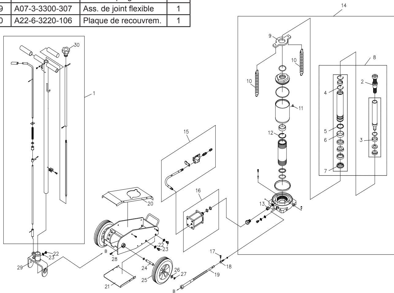
Figure 2 : Illustration des pièces de rechange du modèle 23227
